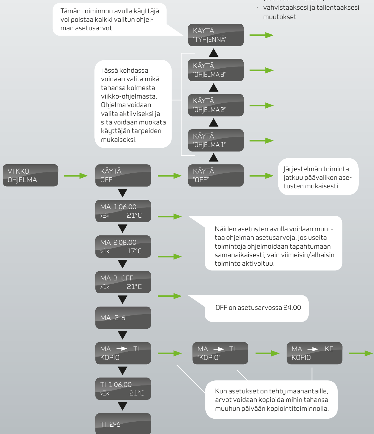
Kuva 11: VIKKO-OHJELMA -valikko
